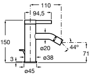
Grifería para bidé Con regulador de chorro a rótula, desagüe automático y enlaces de alimentación flexibles
