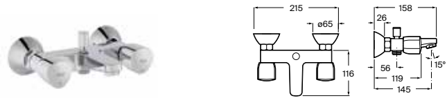
Grifería exterior para baño-ducha Con inversor automático con retención Cromado A5A018EC00 € 122,00
