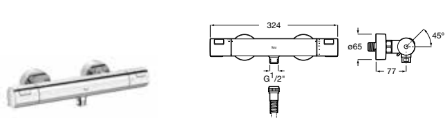
Grifería termostática exterior para ducha Con desviador-regulador de caudal
