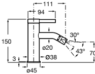
Grifería para bidé con cuerpo liso Con regulador de chorro a rótula y enlaces de alimentación flexibles
