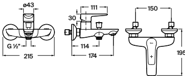
Grifería exterior para baño-ducha Con inversor automático con retención, ducha de mano Natura 80/1, flexible PVC de 1,7 m y soporte articulado
