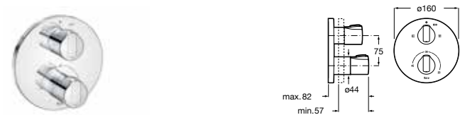
Grifería termostática empotrable para baño-ducha A completar con Roca Box ref. A525869403
