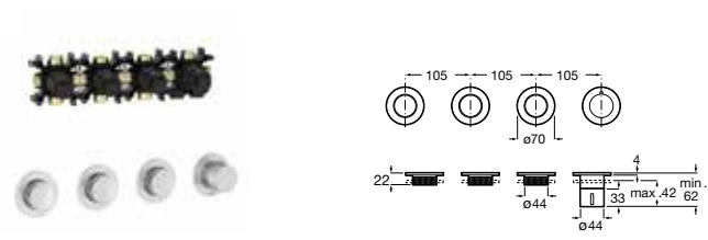
Grifería termostática empotrable 3 vías A completar con cuerpo empotrable
