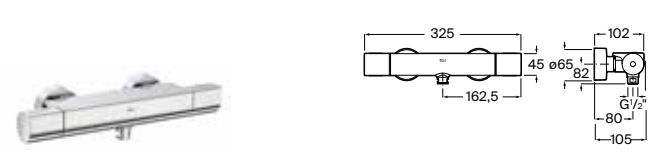
Grifería termostática exterior para ducha
