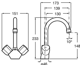
Grifería para lavabo Con aireador, caño giratorio, desagüe automático y enlaces de alimentación flexibles
