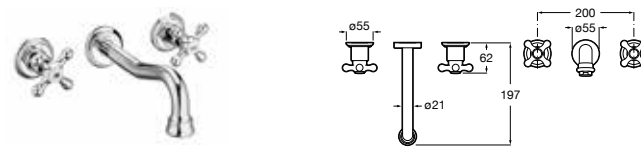
Grifería empotrable para lavabo Cromado A5A474BC00 € 236,00
