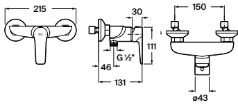
Grifería exterior para ducha Con ducha de mano Natura 80/1, flexible PVC de 1,5 m y soporte articulado
