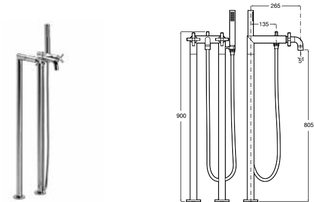
Grifería bimando de pie para baño- ducha Con inversor automático, ducha de mano, flexible de 1,75 m, soporte articulado y columnas verticales de alimentación Cromado A5A2743C00 € 1.416,00
