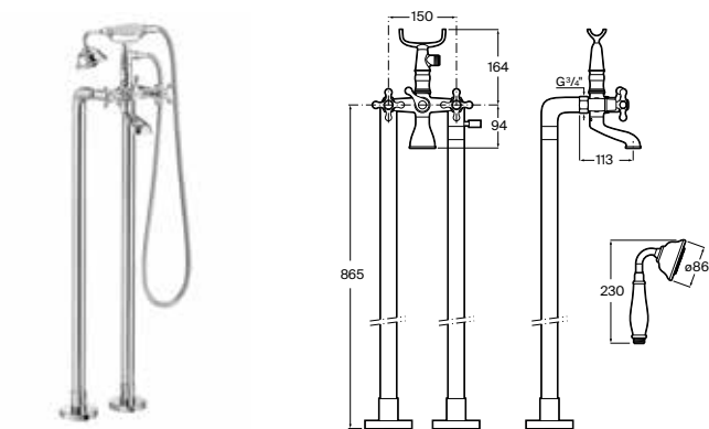
Grifería bimando de pie para baño-ducha Con inversor manual, ducha de mano, flexible de 1,50 m y columnas verticales de alimentación Cromado A5A274BC00 € 639,00
