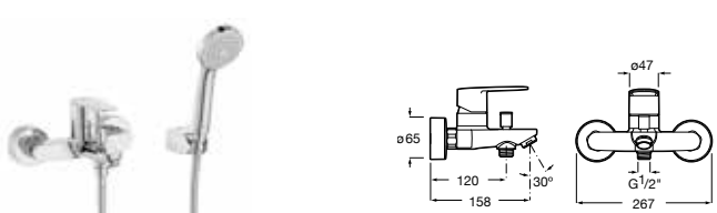
Grifería exterior para baño-ducha Con inversor automático con retención, ducha de mano Natura, flexible de 1,70 m y soporte articulado
