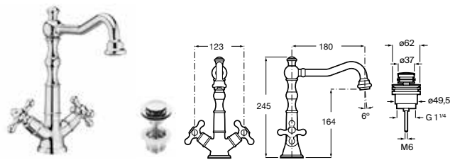
Grifería para lavabo con caño alto y cuerpo liso Con caño alto giratorio, aireador, desagüe click-clack y enlaces de alimentación flexibles Cromado A5A384BC00 € 224,00
