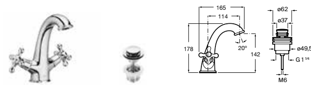
Grifería para lavabo con cuerpo liso Con aireador, desagüe click-clack y enlaces de alimentación flexibles Cromado A5A3A4BC00 € 177,00
