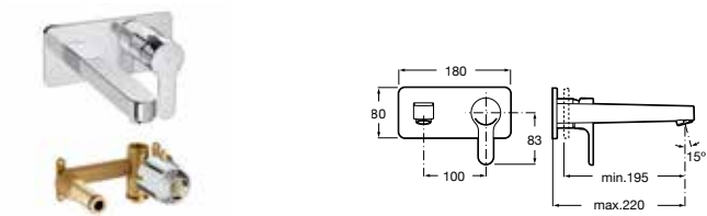
Grifería empotrable para lavabo A completar con cuerpo empotrable universal
