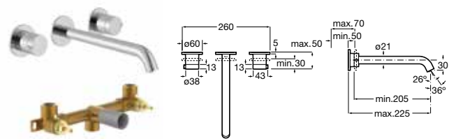
Grifería empotrable para lavabo Longitud de caño 230 mm. A completar con cuerpo empotrable
