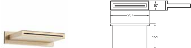
Caño cascada mural con sistema anti cal, Easy Clean
