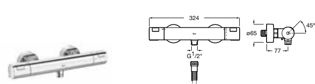
Grifería termostática exterior para ducha
