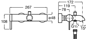
Grifería exterior para baño-ducha Con inversor automático
