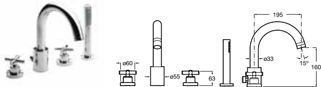
Grifería de repisa para baño- ducha Con caño central alto con inversor, ducha de mano y flexible de 1,75 m Cromado A5A0943C00 € 736,00
