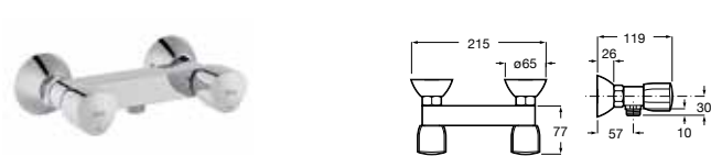
Grifería exterior para ducha Cromado A5A208EC00 € 113,00
