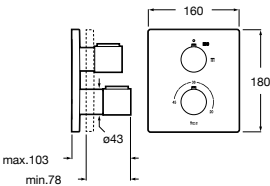
Grifería termostática empotrable para ducha A completar con RocaBox ref. A525869403
