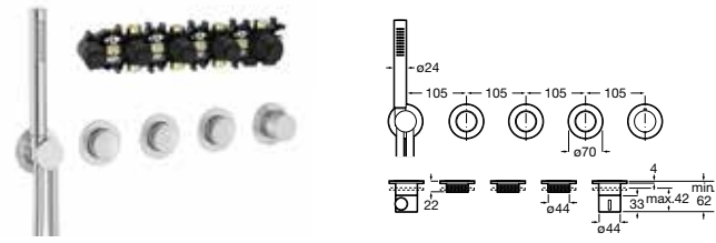
Grifería termostática empotrable 3 vías con ducha de mano y soporte con toma de agua A completar con cuerpo empotrable
