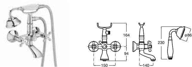
Grifería exterior para baño-ducha Con inversor manual, ducha de mano, flexible de 1,50 m y soporte articulado Cromado A5A014BC00 € 296,00
