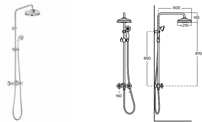
Columna de ducha bimando Con ducha de mano y rociador alto gran caudal Cromado A5A974BC00 € 533,00
