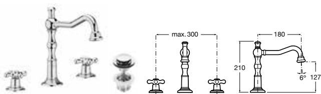
Grifería para lavabo con cuerpo liso Con caño central giratorio, aireador, desagüe click-clack y enlaces alimentación flexibles Cromado A5A444BC00 € 232,00
