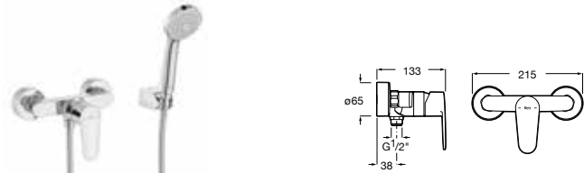
Grifería exterior para ducha Con ducha de mano Natura, flexible de 1,50 m y soporte articulado
