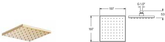
Rociador de techo con sistema anti cal, Easy Clean
