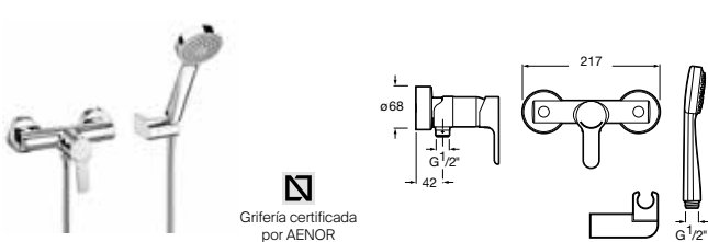
Grifería exterior para ducha Con ducha de mano Stella 80/1, flexible 1,50 m y soporte articulado
