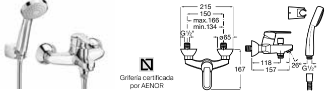
Grifería exterior para baño-ducha Con inversor automático con retención, ducha de mano Natura, flexible de 1,70 m y soporte fijo
