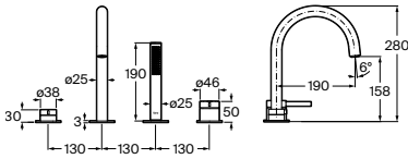
Grifería monomado de repisa para baño-ducha Con caño central, inversor, ducha de mano Stick y flexible de 1,60 m empotrable
