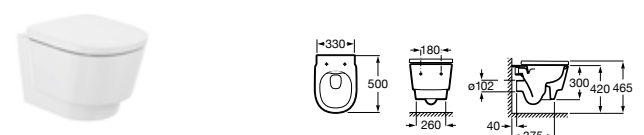
Inodoro suspendido 500 mm de longitud
