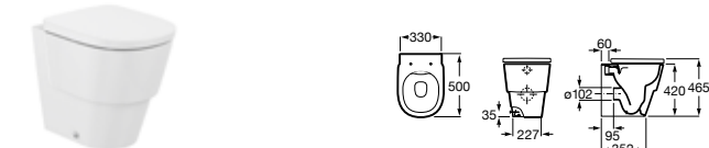
Inodoro de tanque alto o empotrable adosado a pared 500 mm de longitud
