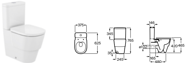
Inodoro de tanque bajo adosado a pared 625 mm de longitud
